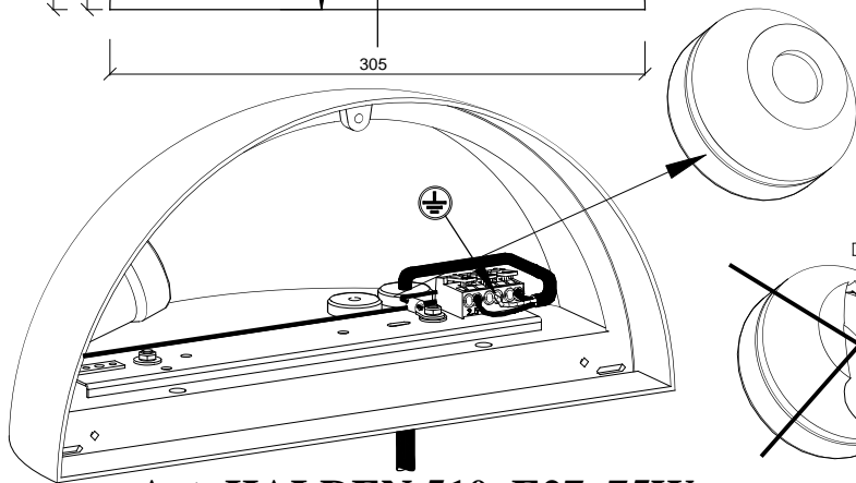
Art. HALDEN 510 E27, 75W
