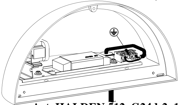
Art. HALDEN 512 G24d-2, 18W Art. HALDEN 514 G24d-3, 26W
